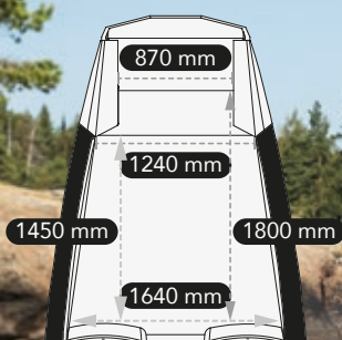
Keulan mitat
