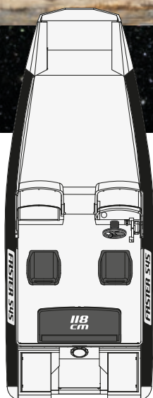
Keulan mitat
