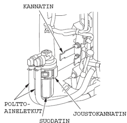
POLTTOAINESUODATIN (vedenerottajan sisäpuolella)
