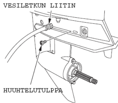
VESILETKUN LIITIN
