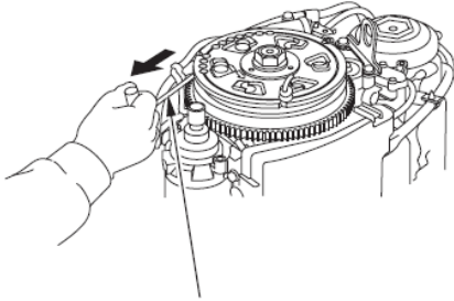
VARAKÄYNNISTYSNARU
